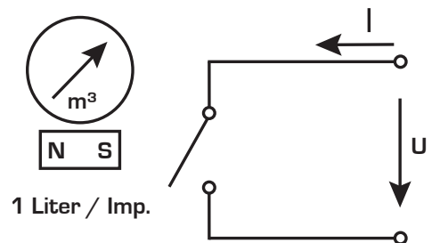
Schaltbild für Kontaktmodul Minomess® Steck pulse 3
