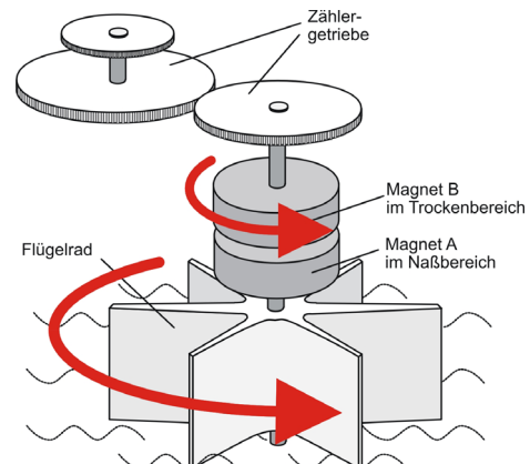
Funktionsprinzip eines Flügelradzählers: Jede Wasserbewegung führt zu einer sichtbaren Bewegung im Wasserzähler.
